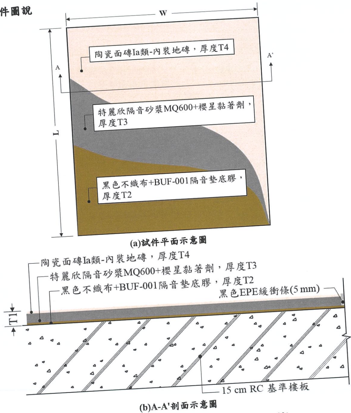
圖5.1 試件平面、剖面示意圖(由委託單位提供)
