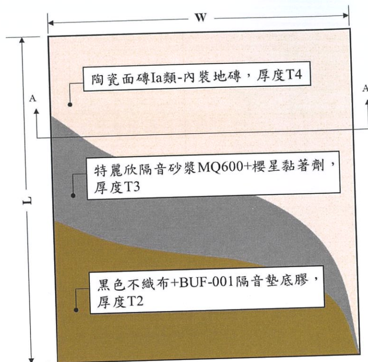
(a)試件平面示意圖
