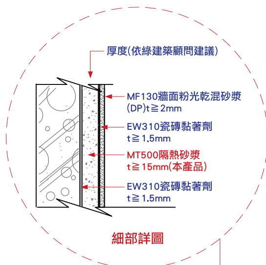
隔熱砂漿施工大樣圖
